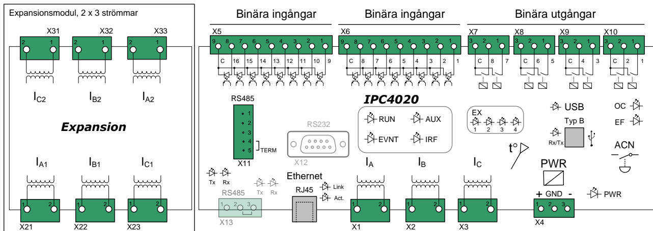
Figur 1. Översikt IPC4020 med expensionsenhet för två extra detektorfunktioner (till vänster). Utgångarna på kontakterna X8 och X10 är anslutna till kraftigare reläer.
